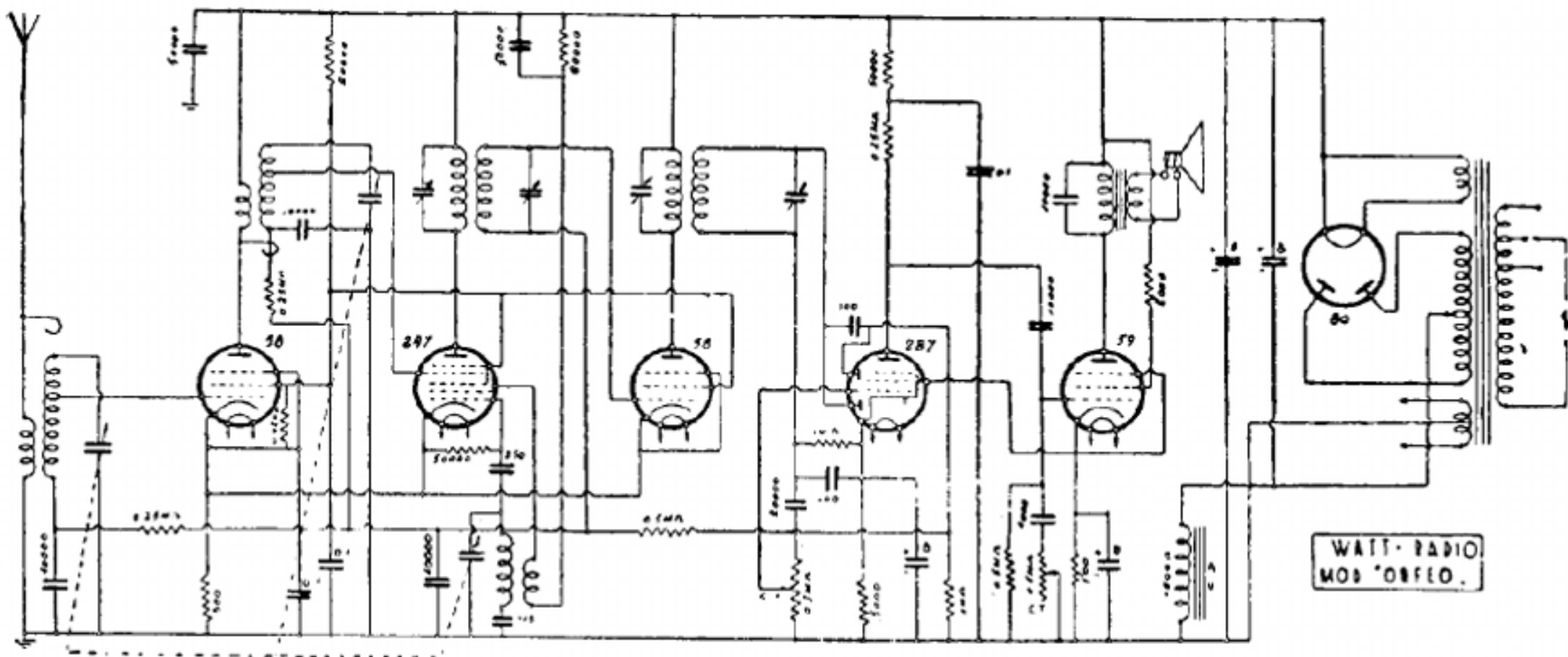
WATT RADIO. — Modello « Orfeo ». • Produzione 1933. • Media frequenza: 125 kc.
